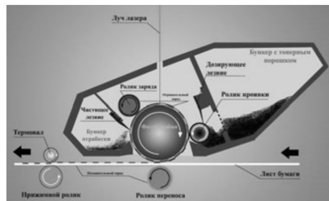
Схема работы электрофотографического печатающего устройства.
